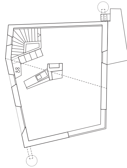
DACHGESCHOSS_ATTIC FLOOR
