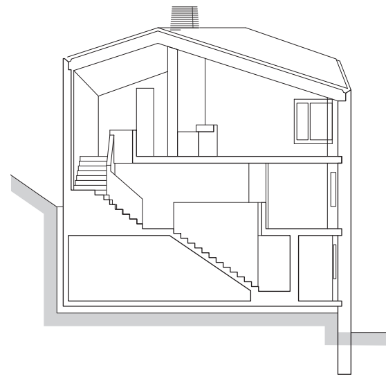
SCHNITT_SECTION
